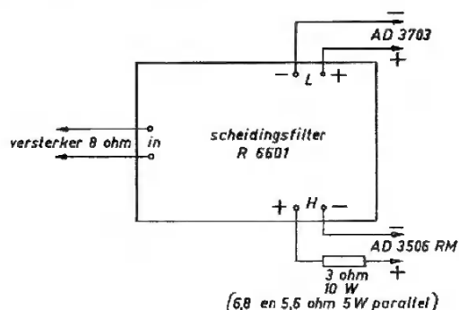
Aansluiting van het scheidingsfilter
